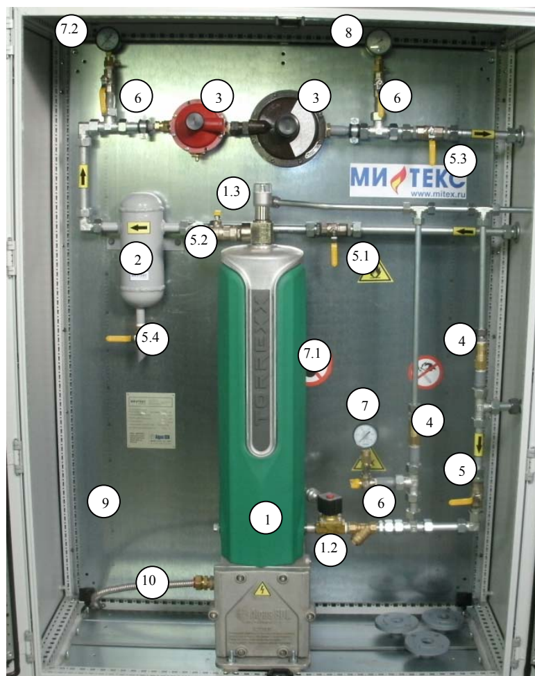
Устройство испарительной установки Рис.1
